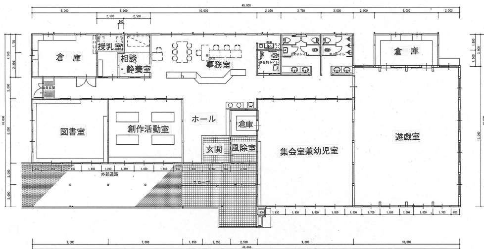
平面図 S:1/200
