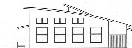
東側立面図
