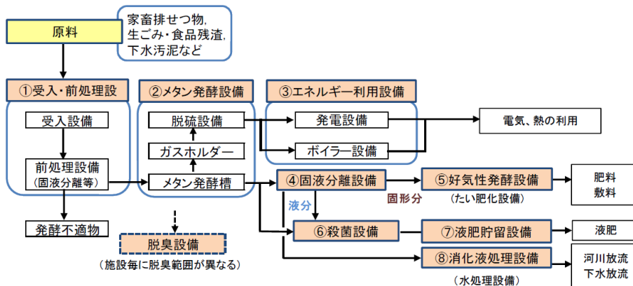
メタン発酵施設を構成する設備
