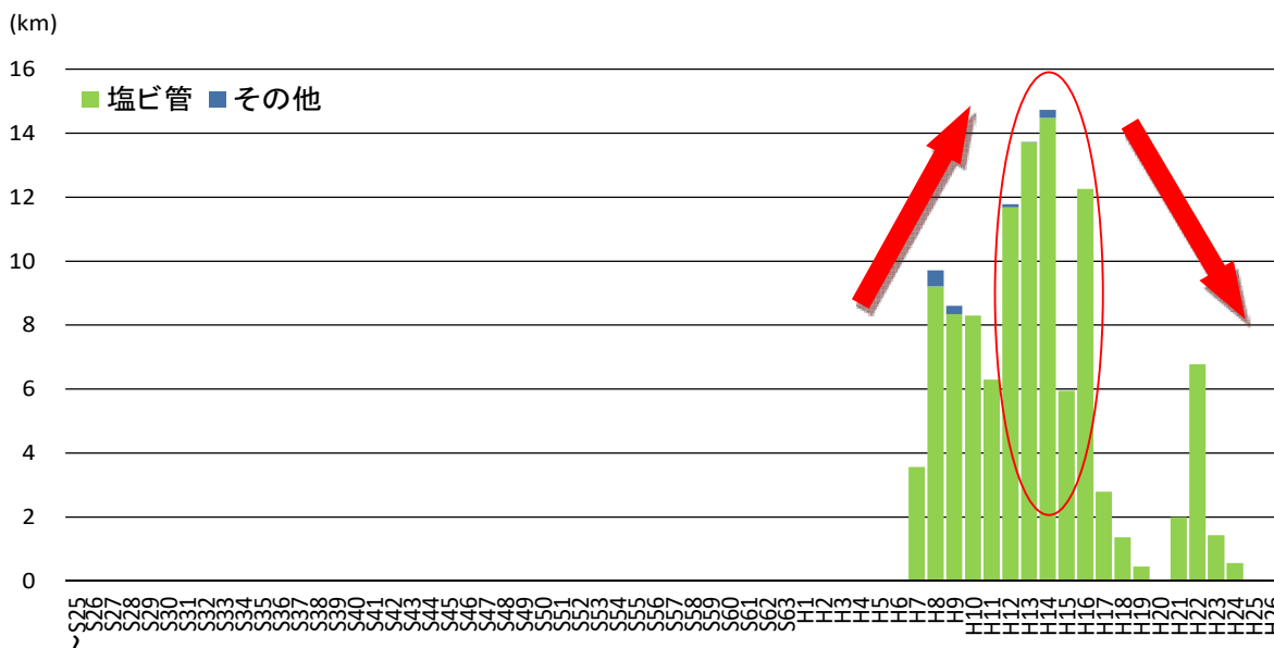
図 2-26 集落排水(管渠)の年度別整備延長の推移
