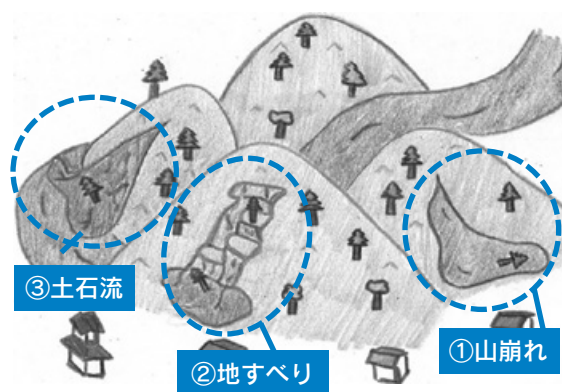
図1 山地災害の発生形態
