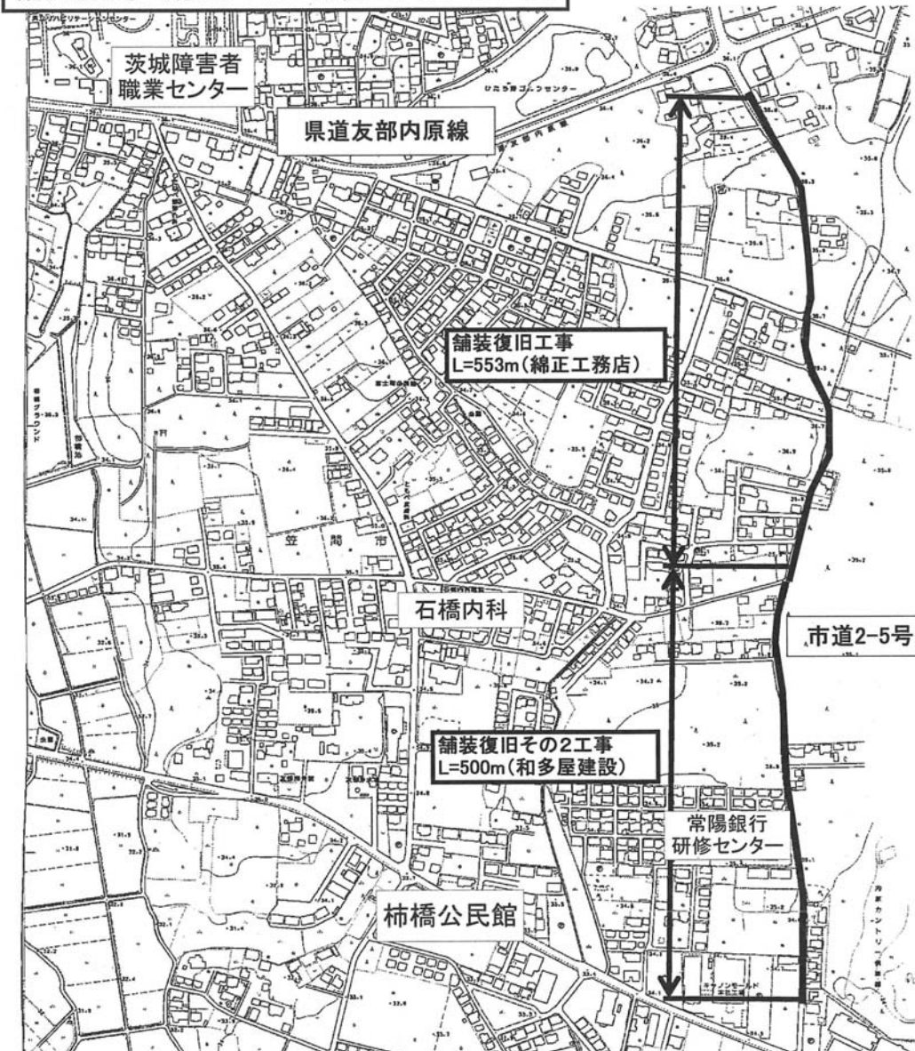
霞ヶ浦用水3期地区 H22舗装工事施工位置図
